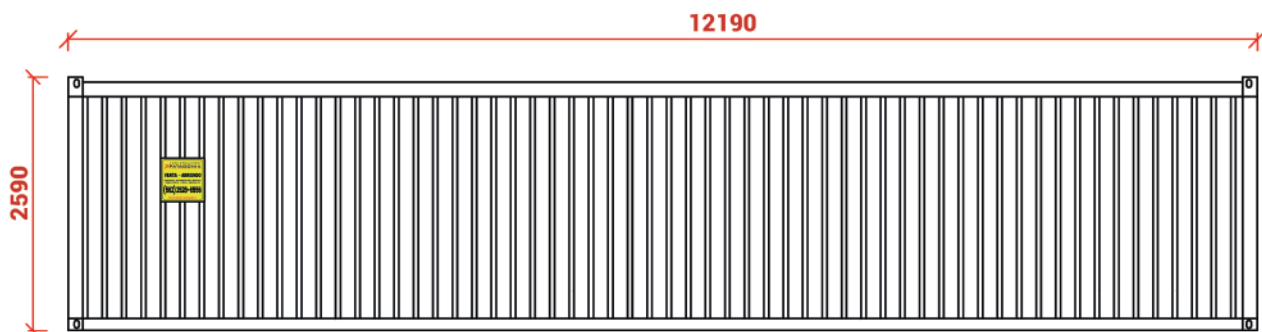
Elevación Sur
