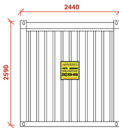
Elevación Oeste
