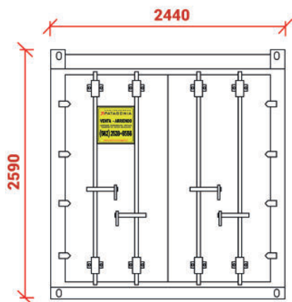
Elevación Este
