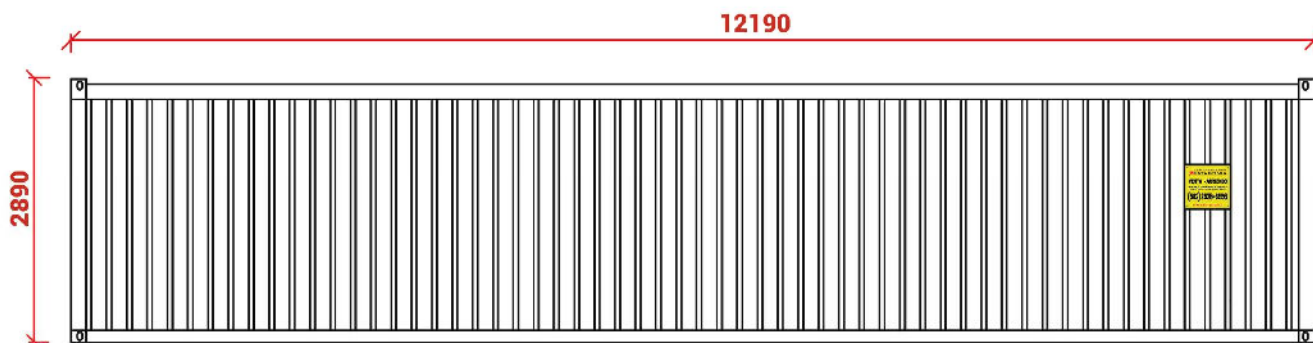
Elevación Norte
