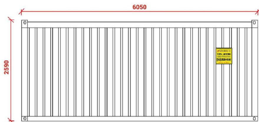
Elevación Norte
