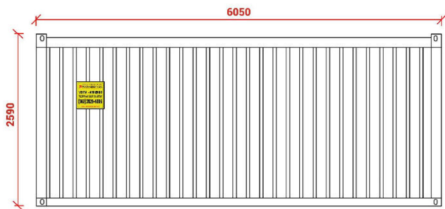
Elevación Sur
