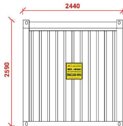
Elevación Oeste
