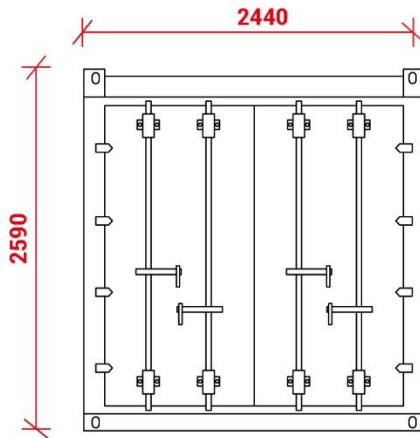
Elevación Este
