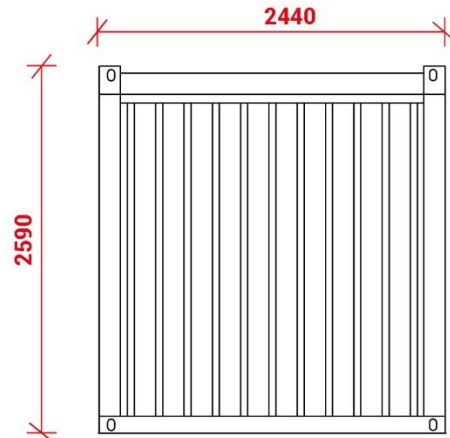
Elevación Oeste
